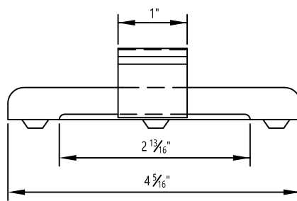
NedZink® Standing Seam Sliding Clip
