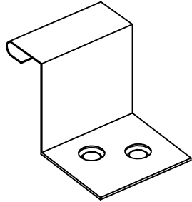
NedZink® Standing Seam Fixed Clip
