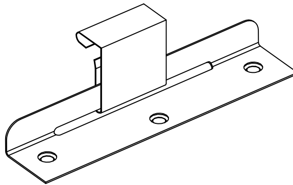
NedZink® Standing Seam Sliding Clip
