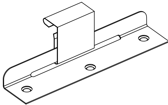
NedZink® Standing Seam Sliding Clip
