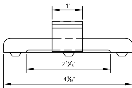
NedZink® Standing Seam Sliding Clip
